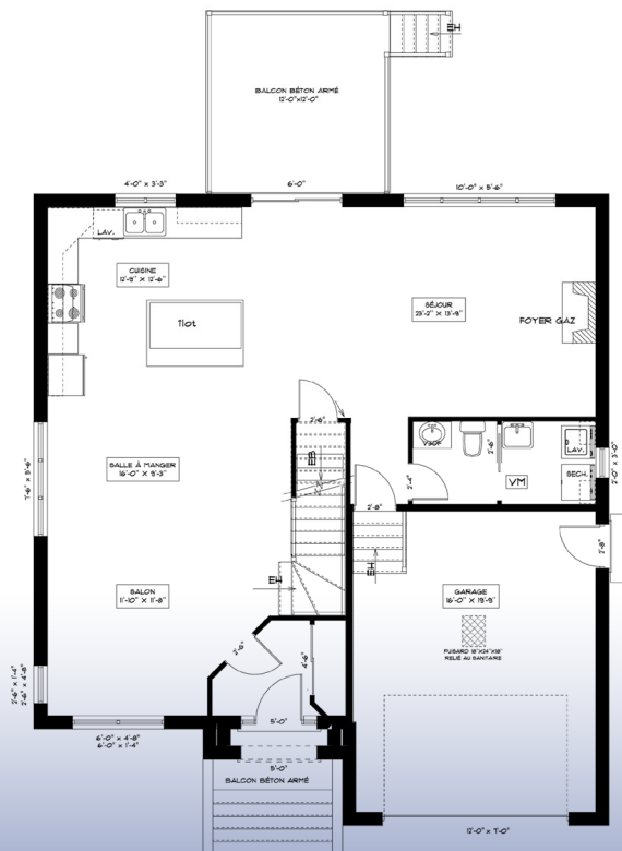
REZ DE CHAUSSÉE (1121.3 p.c.)
